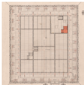
昭和実測図 名古屋城天守初層平面図
