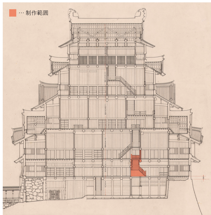
昭和実測図 名古屋城天守縦断面図
