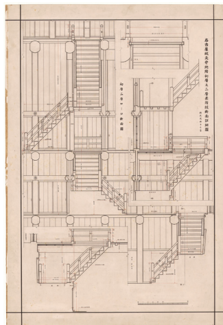
昭和実測図 名古屋城天守地階初層及二層表階段断面詳細図
